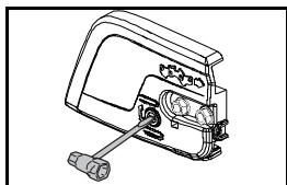
Tensión de la cadena: modelos de ajuste lateral
